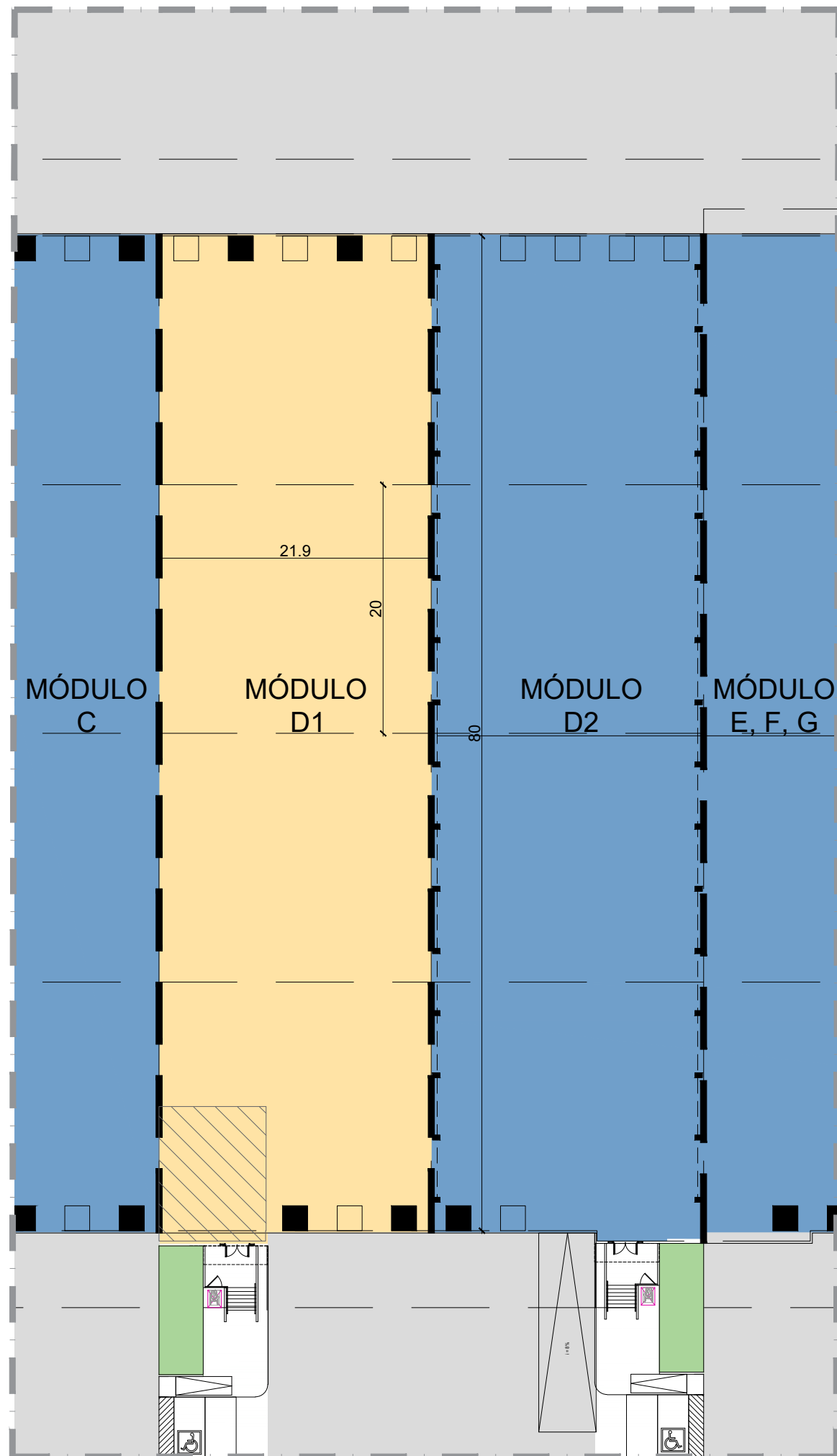
PLANTA - MODULO D1
