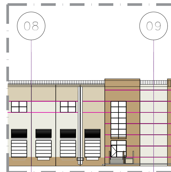
DETALHE - ELEVACÃO
