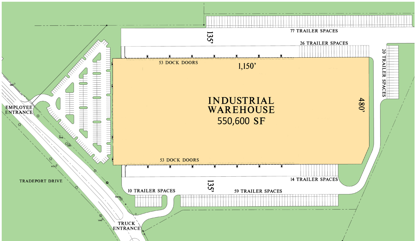
T-40 550,600 SF SITE PLAN OPTION
